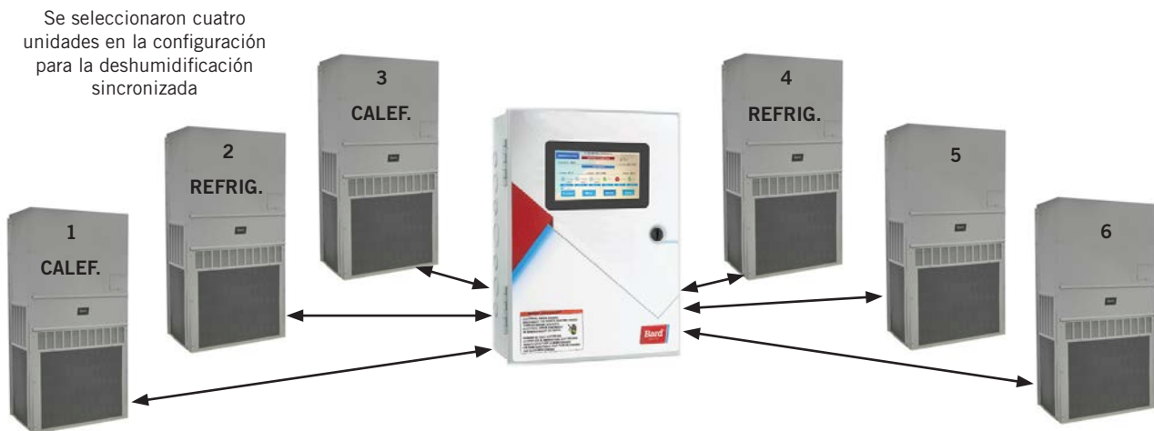
FIGURA 7 Deshumidificación sincronizada
