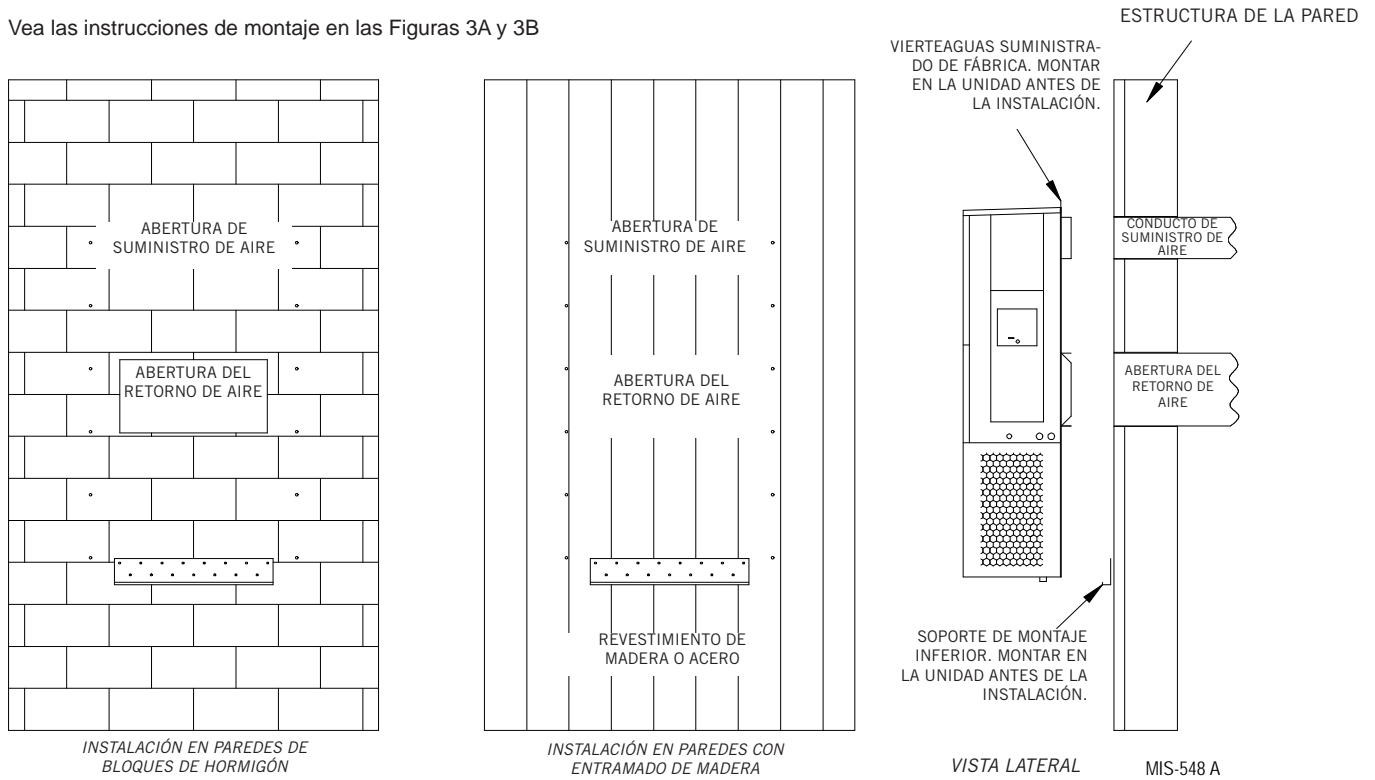
FIGURA 5 Instrucciones para montaje en pared
