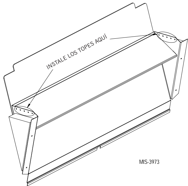
FIGURA 1 Compuerta reguladora de aire fresco
