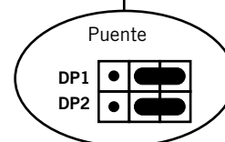
Posición del puente para 0-1 Vcc
