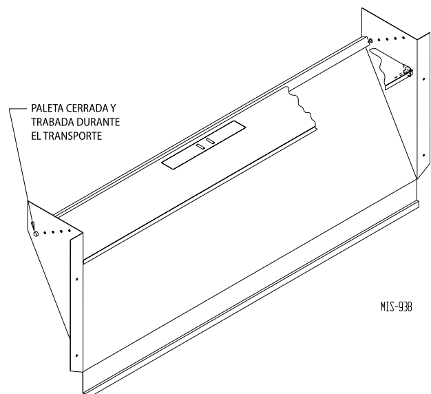
FIGURA 1 Regulador de aire exterior
